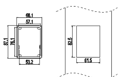
Рисунок 4-14. Настенное крепление
